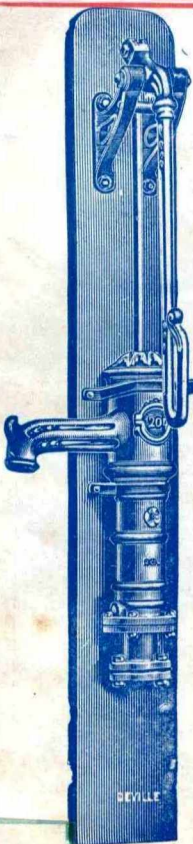
POMPES DES ARDENNES" à balancier de face ou côté, avec ou sans aiguille Nos 200 à 212
