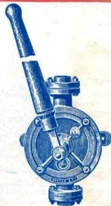
POMPES DEMI-ROTATIVES Nos 0-1-2-3-4-5-6-7-8 aspirantes et foulantes, à double et quadruple effet
